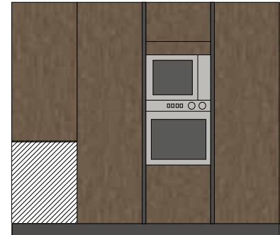
PROSPETTO COLONNE
